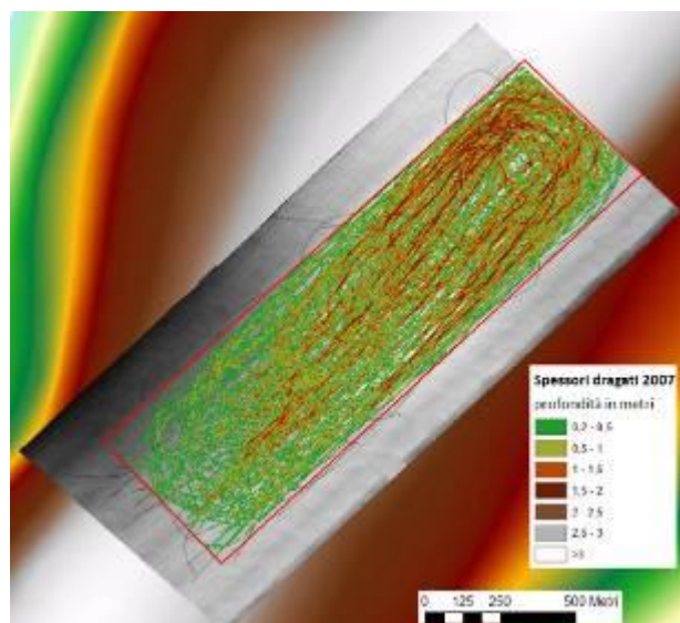
Figura IV.4.4.2.2 Calcolo degli spessori dragati nel 2007 nell'area C1
